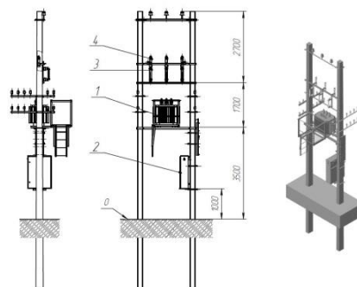
1. Трансформатор 2. Щит РЩТ 3. Бисимбиольный предохранитель 4. Ограничитель перенапряжения (вентильный разрядник)
